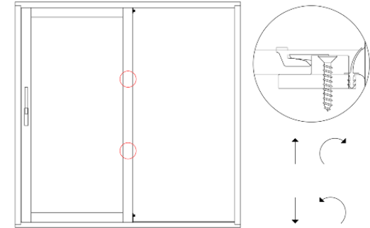
Kuva 4. Tarkista välilukon toiminta. Säädä tarvittaessa Torx 20 avaimella tiivistettä raottamalla. Myötäpäivään pyörittämällä puitteen puristus keskitolppaan löystyy.
